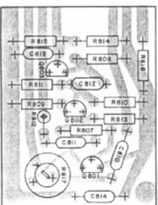
IF Xtal Oscillator 1P84306A43
